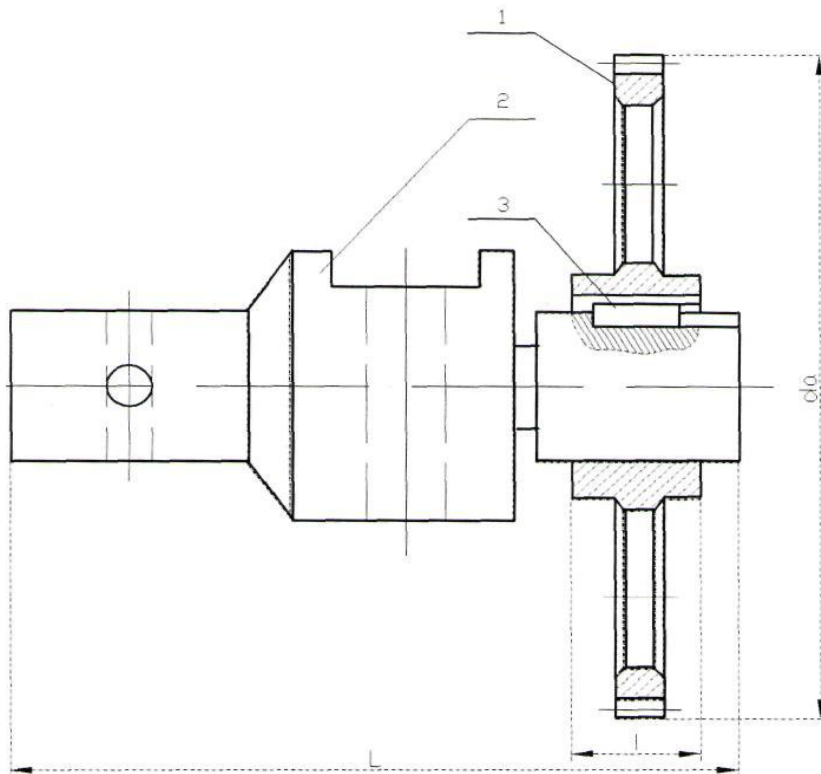
1 - зубчатое колесо; 2 - вал; 3 - шпонка.
