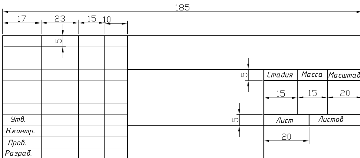
Рисунок И.6 - Основная надпись для первого листа строительного изделия
