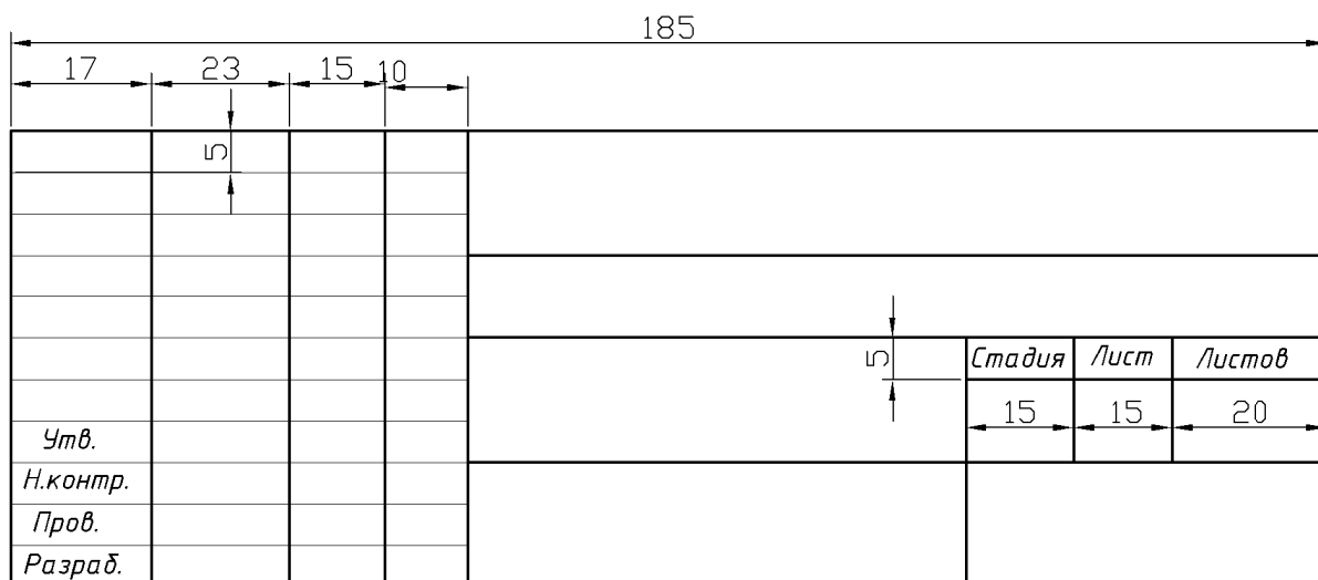
Рисунок И.5 - Основная надпись для листов основного комплекта рабочих чертежей зданий и сооружений
