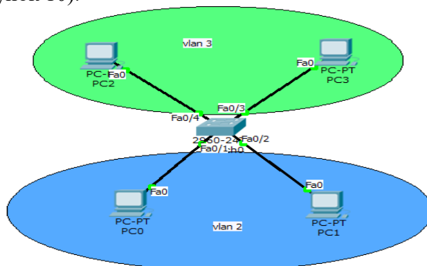
Рисунок 10- Соединение устройств
