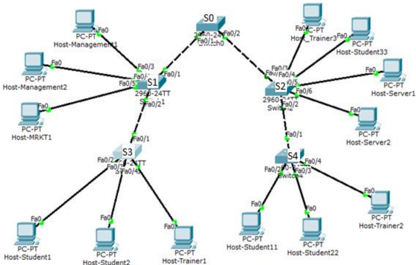
Рис. 1 Топология сети
