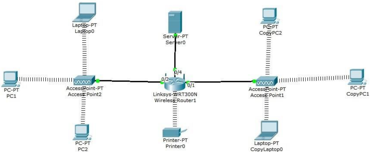
Рис.2.1 Схема сети
