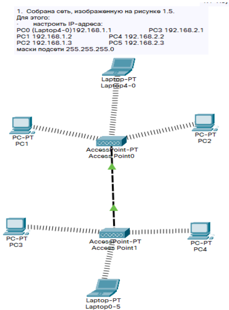
Рисунок 1.5 – пример телекоммуникационной сети
