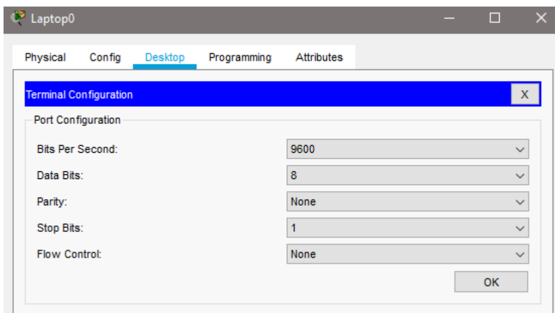
Рис. 5 – Вход в терминал для настройки коммутатора через консоль
