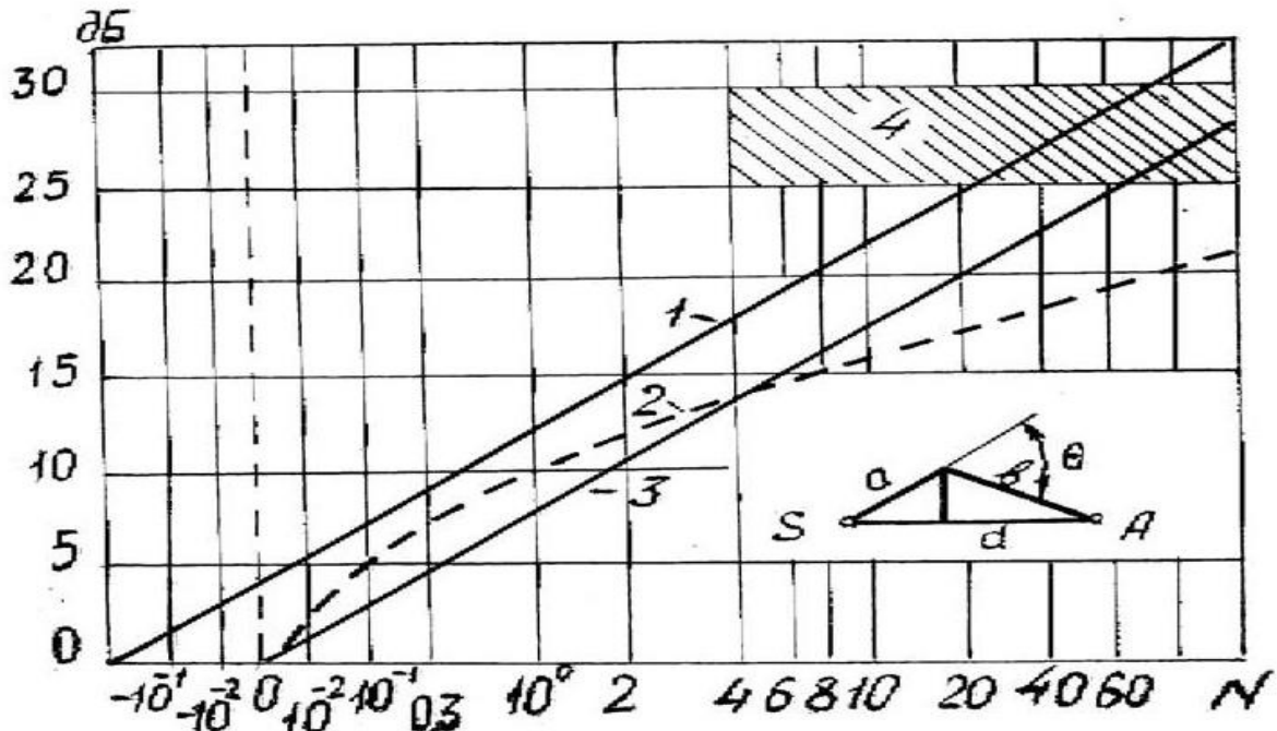
Рис.1. Зависимость снижения уровня звукового давления от числа Френеля S - источник звука; A - точка наблюдения; 1 - точечный источник высоко над землей; 2 - линейный источник; 3 - точечный источник на земле; 4 - область максимально достижимого снижения; ? - теневой угол;
