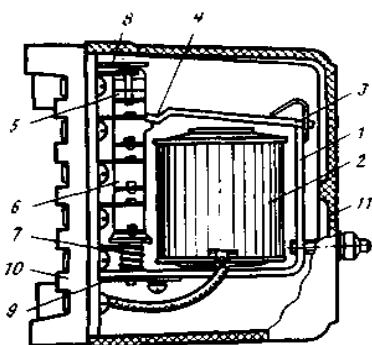
Рис. 2.13. Промежуточное реле типа РП-23
