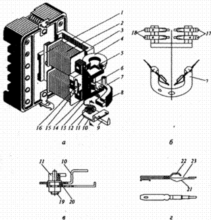
Рис. 2. Общий вид реле РТ40 (РН50): а — конструкция реле; б — изоляционная колодка с неподвижными контактами; в — регулировочный узел; г — контактный узел; 1 — сердечник; 2 — каркас с обмоткой; 3 — алюминиевая стойка; 4 — демпфер; 5 — верхняя полюсь; 6 — подвижной контакт; 7 — изоляционная колодка; 8 — шкала уставок; 9 — указатель уставки; 10 — пружинодержатель; 11 — шестигранная втулка; 12 — спиральная пружина; 13 — хвостовик; 14 — якорь; 15 — фасонная пластинка; 16 — левый упор; 17 — правая пара неподвижных контактов; 18 — левая пара неподвижных контактов; 19 — фасонный винт; 20 — пружинящая шайба; 21 — задний гибкий упор; 22 — передний упор; 23 — бронзовая пластинка с серебряной полоской
