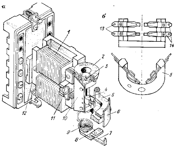
Рисунок 2 общий вид реле напряжения РН - 50
