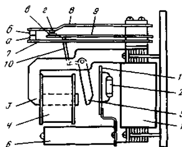
Рис. 2.14. Устройство промежуточного реле типа РП-341:
