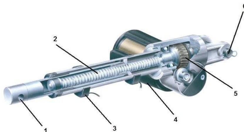
Рисунок 1 Устройство электропривода 1 — Передний крепеж; 2 — Винтовая передача; 3 — Концевой датчик; 4 — Электродвигатель; 5 — Зубчатая передача; 6 — Задний крепеж
